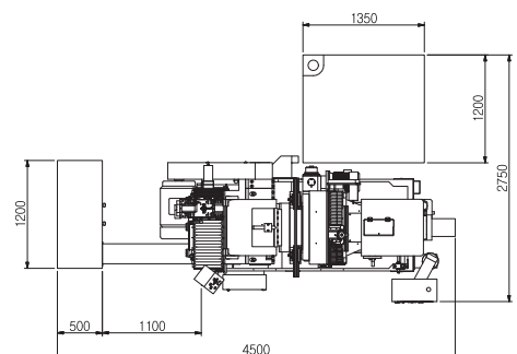
HCG-400 CNC
